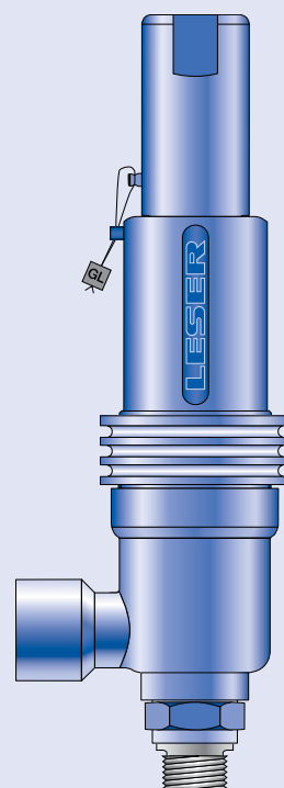
Тип 459 Колпак H2 С уравнивающим сильфоном
