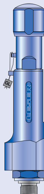
Тип 437 с наружной резьбой Корпус выпускной части 1/2" Герметичная головка H4 Удлиненная версия
