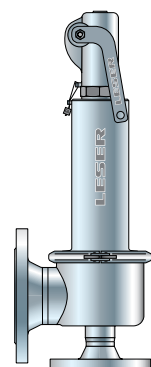
Тип 444 Герметичный рычаг H4 Закрытый кожух Стандартная конструкция
