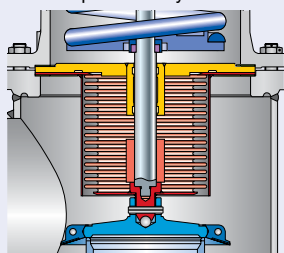
Сиффон из нержавеющей стали J68: Открытый кожух J78: Закрытый кожух
