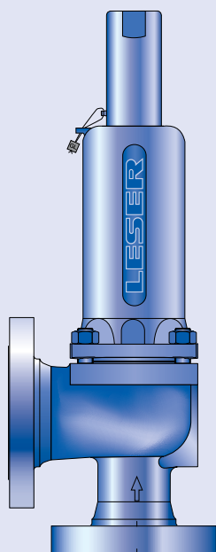
Тип 441 Колпак H2 Закрытый кожух Стандартная конструкция
