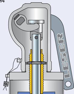
Герметичный рычаг H4 H4
