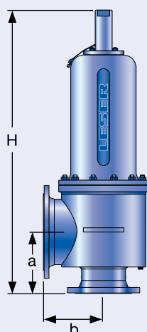
Конструкция стандартная и с уравнивающим сильфоном
