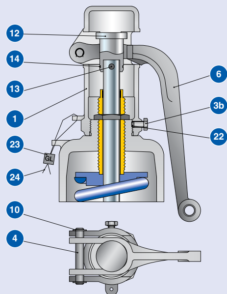
Рычаг подрыва Н3
