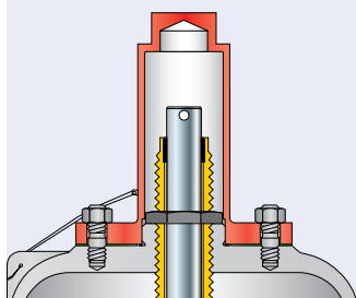
Винт-блокиратор J69: Рычаг Н6 с фланцевым соединением J70: Колпак Н1 с фланцевым соединением
