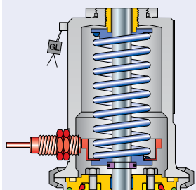
Индикатор подъема в кожухе J38: Переходник кожуха Dy25 J93: Индикатор подъема
