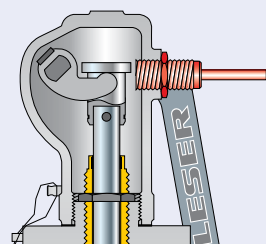
Индикатор подъема H4 От Dy 40 до Dy 80 J38: Переходник H4 J93: Индикатор подъема
