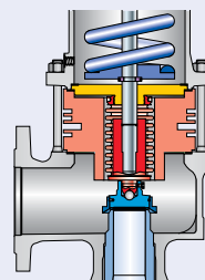
Комплект для переоборудования с установкой сиффона из нержавеющей стали по заявке
