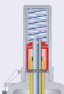
Кольцевой амортизатор H2 J65
