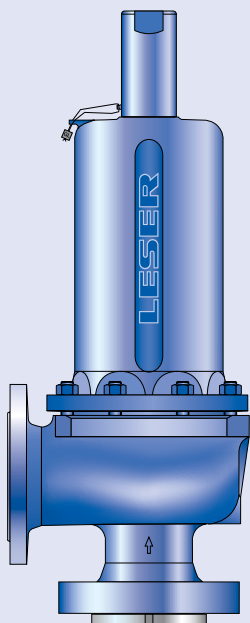
Тип 458 Колпак H2 Закрытый кожух Стандартная конструкция
