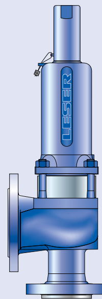
Тип 441 со сплошным соплом Колпак Н2 Закрытый кожух Конструкция с уравновешивающим сильфоном
