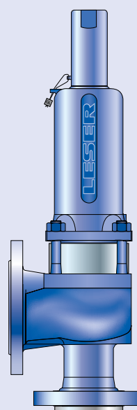
Тип 441 со сплошным соплом Колпак H2 Закрытый кожух Конструкция с уравнивающим сифоном
