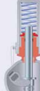
Кольцевой амортизатор H4 J66
