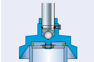
Герметичный колпак H2 H2
