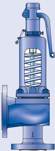
Type 442 Со сплошным соплом Рычаг подрыва Н3 Открытый кожух Стандартная конструкция
