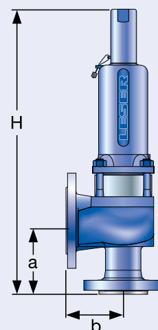
Конструкция с уравнивающим сильфоном
