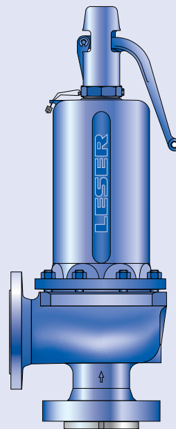
Тип 458 Рычаг подрыва H3 Закрытый кожух Стандартная конструкция
