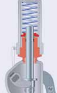
Кольцевой амортизатор H4 J66
