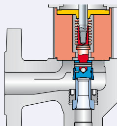
Комплект для переоборудования с установкой уравновешивающего сифона Арт. №, см. стр. 02/14
