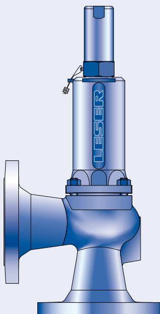
Тип 433 Колпак H2 Закрытый кожух Стандартная конструкция
