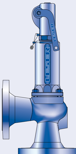
Тип 433 Герметичный рычаг H4 Закрытый кожух Стандартная конструкция
