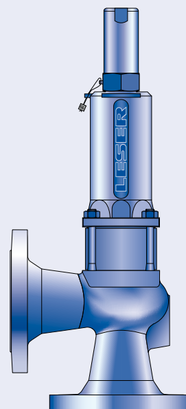
Тип 433 Колпак H2 Закрытый кожух Конструкция с уравнивающим сифоном
