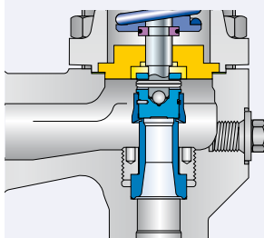
Уравновешивающий сифон J68: Открытый кожух J78: Закрытый кожух
